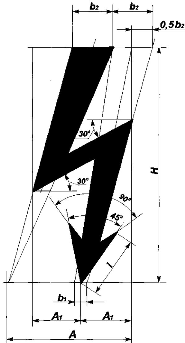
Рисунок Н.1 — Графический символ электрического напряжения
